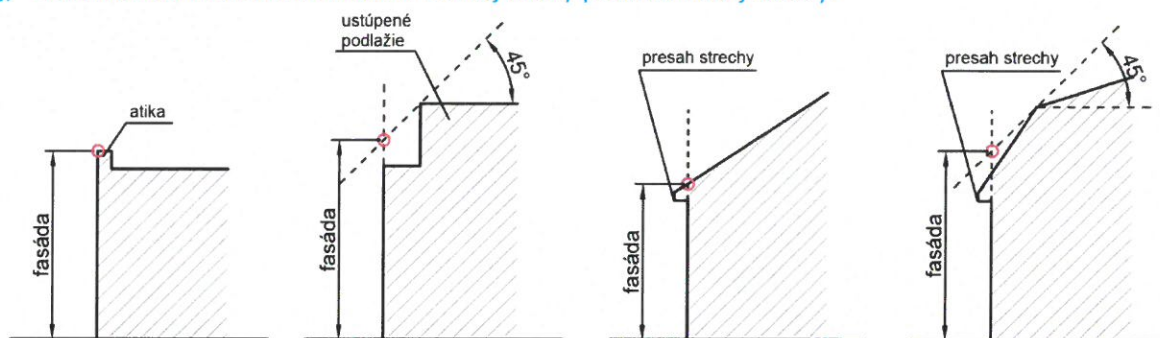
určenie hornej hrany posudzovanej fasády
