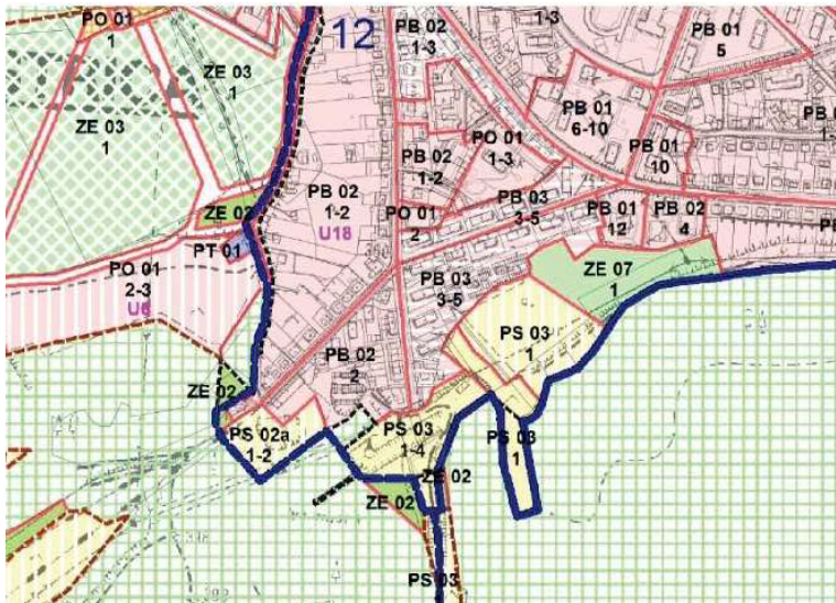
VÝKRES č.7a REGULATÍVY FUNKČNÉHO VYUŽÍVANIA A PRIESTOROVÉHO USPORIADANIA ÚZEMIA - FUNKČNÉ A VÝŠKOVÉ REGULATÍVY VÝREZ Z PLATNÉHO ÚPN M BANSKÁ BYSTRICA
