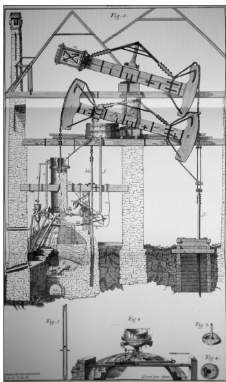
Nákres Potterovho ohňového stroja
